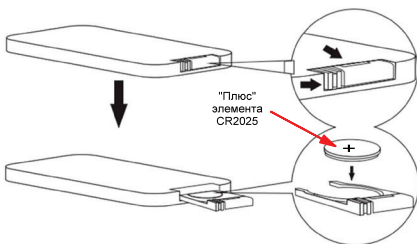
Рис.2. Установка элемента питания.
