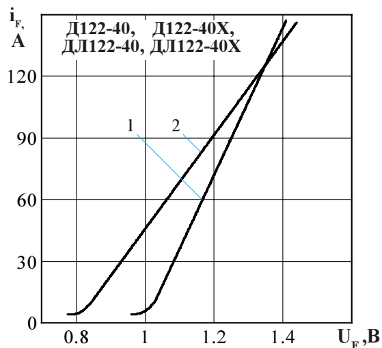
Рисунок 1 - Предельная прямая вольтамперная характеристика при температуре перехода 25 °C (1) и максимальной температуре перехода T_{жм} (2) I_F = 3,14 I_{F(AV)}
