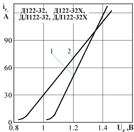
Рисунок 1 - Предельная прямая вольтамперная характеристика при температуре перехода 25 °C (1) и максимальной температуре перехода T_{жм} (2) I_F = 3,14 I_{F(AV)}
