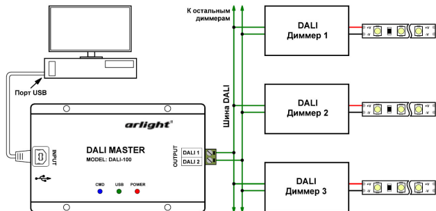
Рис.1. Схема соединения оборудования.
