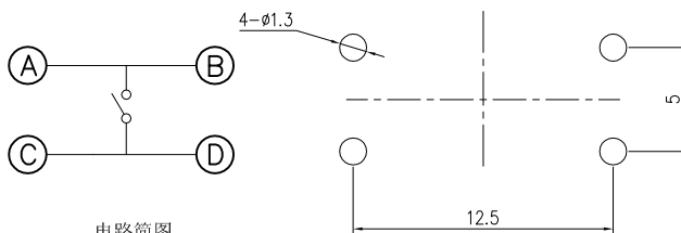
印制线路板 Recommended P.C.B layout
