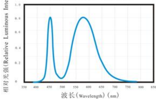
光谱分布特性曲线 Relative Spectral Distribution
