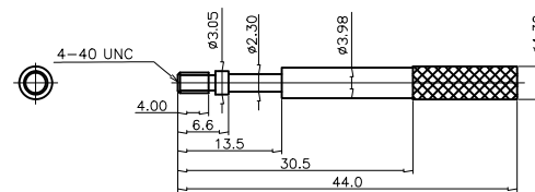
Long BOLT
