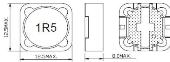
DIMENSIONS(mm) 外型尺寸
