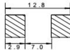
LAND PATTERNS(mm) 焊盘尺寸
