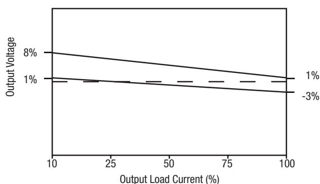
15V Output
