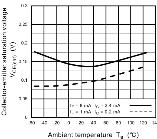
Fig. 11.10 V_{CE(sat)} - T_a
